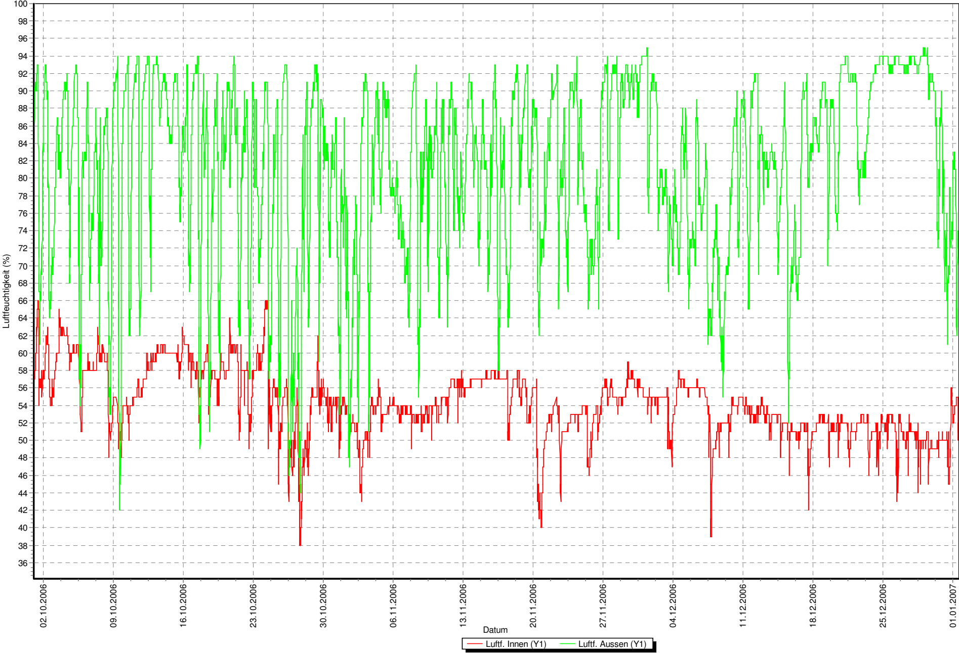
Luftfeuchtigkeit-Diagramm 2006
